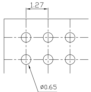
P.C.B Hole Layout
