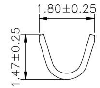
SEC:B-B
